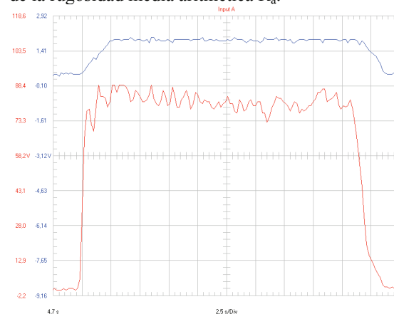
Figura 4: Gráficos tipo de M_t (arriba) y F_a registrados por el osciloscopio.
