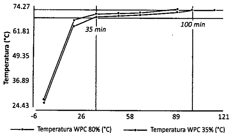
Gráfico 1 - Curva de calentamiento de las mezclas WPC 35% y 80%.
