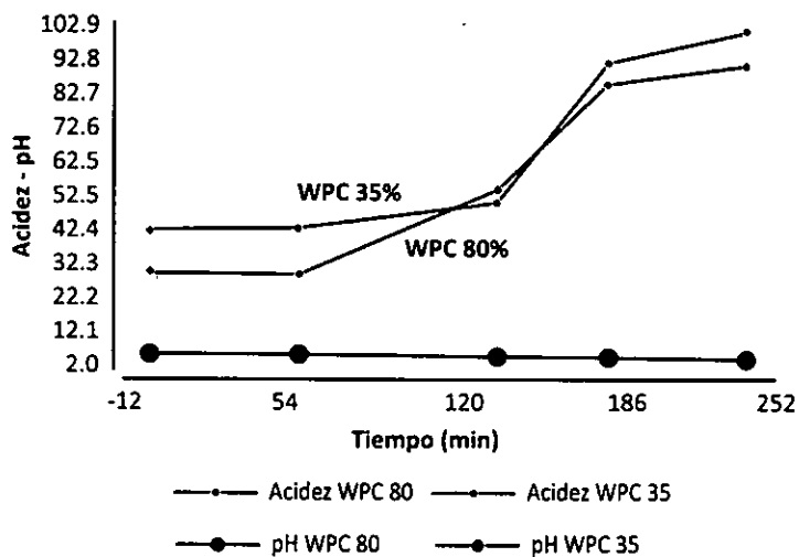
Gráfico 2 - Curva de fermentación de yogur con WPC 35% y 80%
