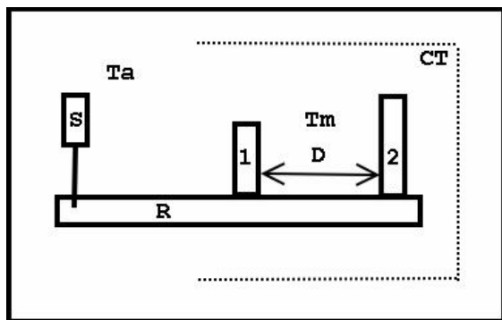
Fig. 1: Esquema del sistema. (S) Transductor ultrasónico. (R) Riel de soporte. (CT) Cámara térmica. (1) Primer obstáculo. (2) Segundo obstáculo. (D) Distancia entre obstáculos. (Ta) Temperatura ambiente. (Tm) Temperatura medida.
