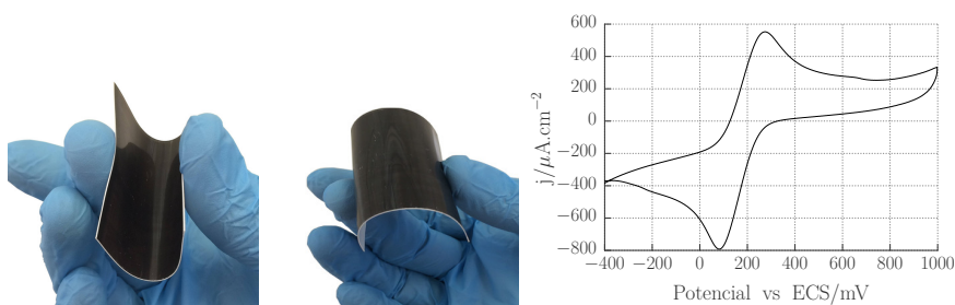
Figura 6.3: Electrodo basado en nanotubos de carbono impresos por inyección de tinta en donde se muestra la flexibilidad de la tinta y su respuesta electroquímica con una sonda de FeCN 2,5 mM en solución de KCl 100 mM a 50 \text{ mV s}^{-1} .
