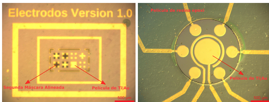
a. Alineación de la segunda máscara con la película de Ti|Au ya depositada.
