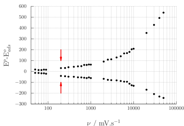
Figura 4.12: Desplazamiento de los potenciales en función de la velocidad de barrido. Las flechas rojas indican la velocidad característica para el cambio de régimen, de capa delgada a control difusional.
