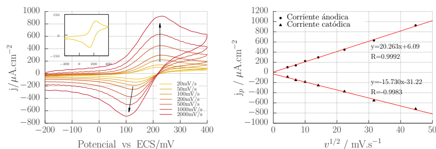
a. Voltamogramas a diferentes velocidades de barrido para FcOH 1 mM. Recuadro: VC para una velocidad de barrido de 20 mV s -1 .
