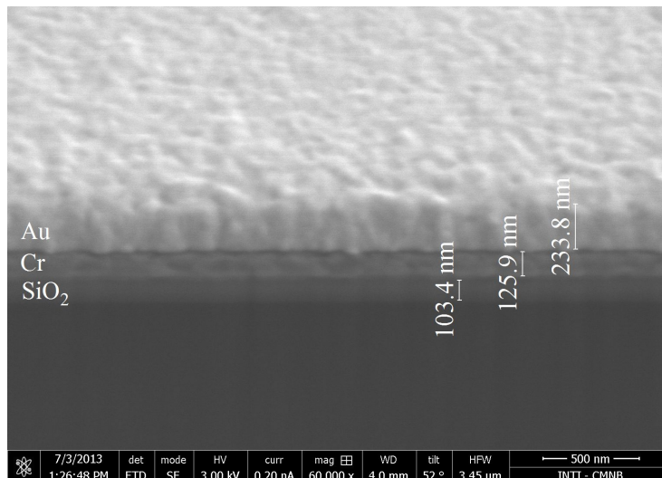
Figura 5.8: Corte transversal de los electrodos, donde se observan detalles de la bicapa Cr|Au depositada sobre una oblea de silicio con un depósito aislante de SiO 2 .
