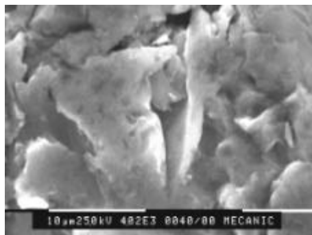
Fig. 4 Micrografía electrónica de la muestra G0 tratada con blasting .
