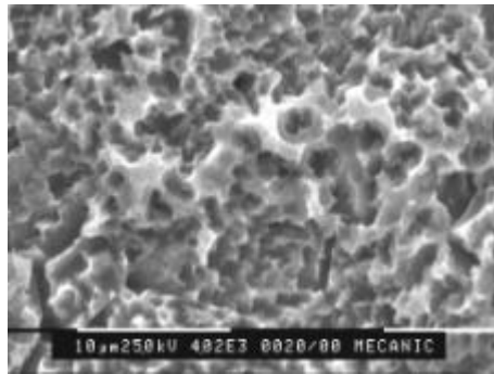
Fig. 3 Micrografía electrónica de la muestra D6 desbastada y luego atacada con HCl 9M.
