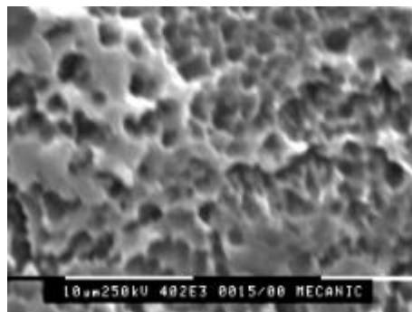
Fig. 2 Micrografía electrónica de la muestra D2 desbastada y luego atacada con \text{H}_2\text{SO}_4 9M.
