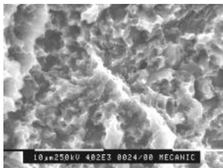
Fig. 6 Imagen SEM de la muestra G6 tratada con blasting y luego atacada con HCl 9M.
