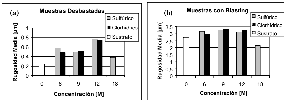
Fig. 7 Rugosidad media del sustrato y de las muestras atacadas (a) con desbaste mecánico (b) con tratamiento de blasting .
