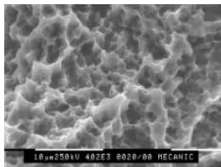
Fig. 5 Imagen SEM de la muestra G2 tratada con blasting y luego atacada con H 2 SO 4 9M.
