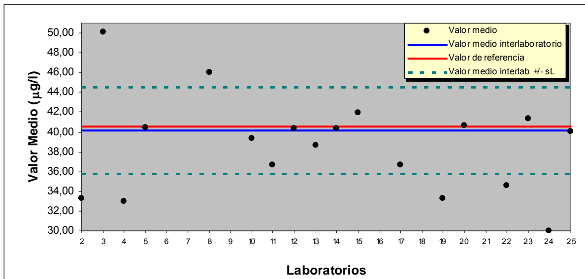
GRÁFICO 3 Datos enviados por los participantes – Cromo
