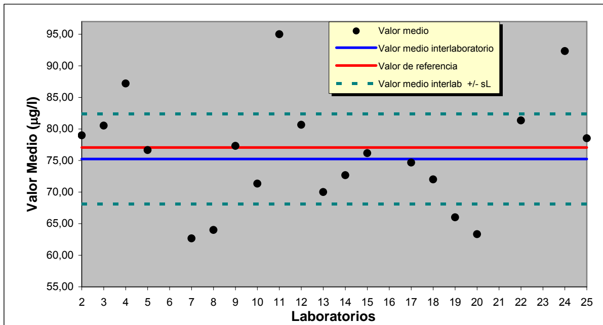
GRÁFICO 5 Datos enviados por los participantes – Plomo
