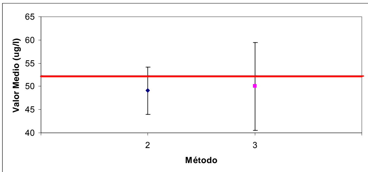
GRÁFICO 11 Desviación según método - Arsénico
