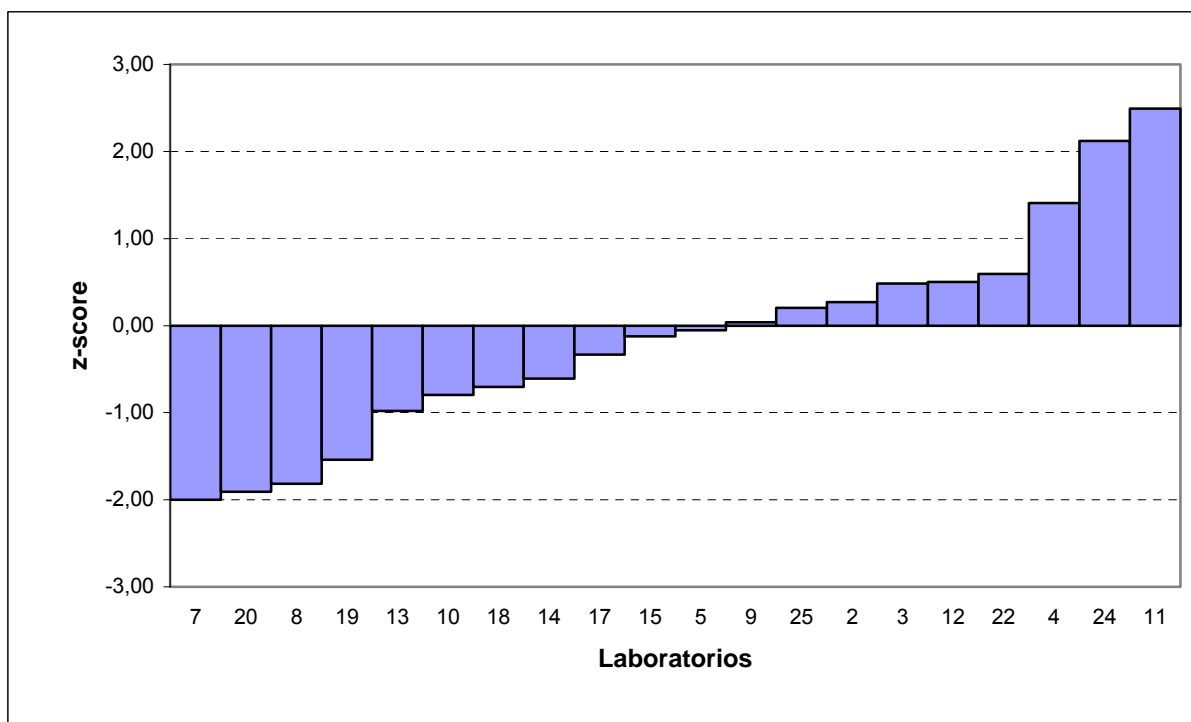
GRÁFICO 10 Parámetro z – Plomo
