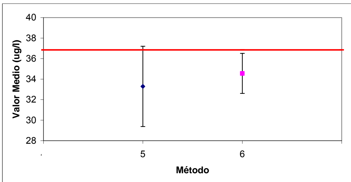
GRÁFICO 12 Desviación según método – Cadmio
