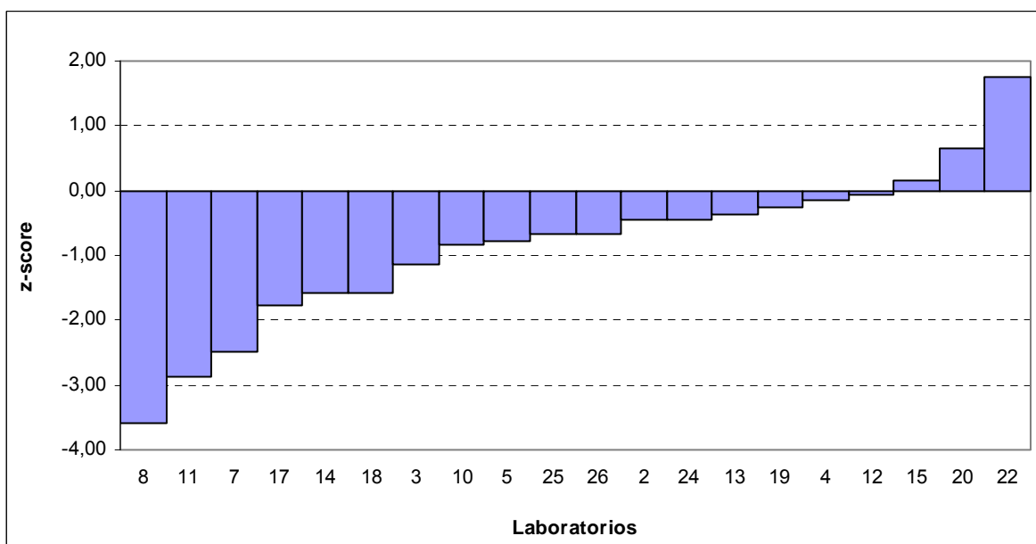
GRÁFICO 7 Parámetro z –Cadmio
