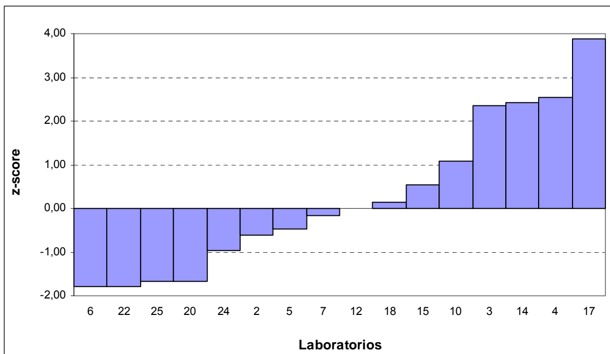
GRÁFICO 9 Parámetro z – Mercurio
