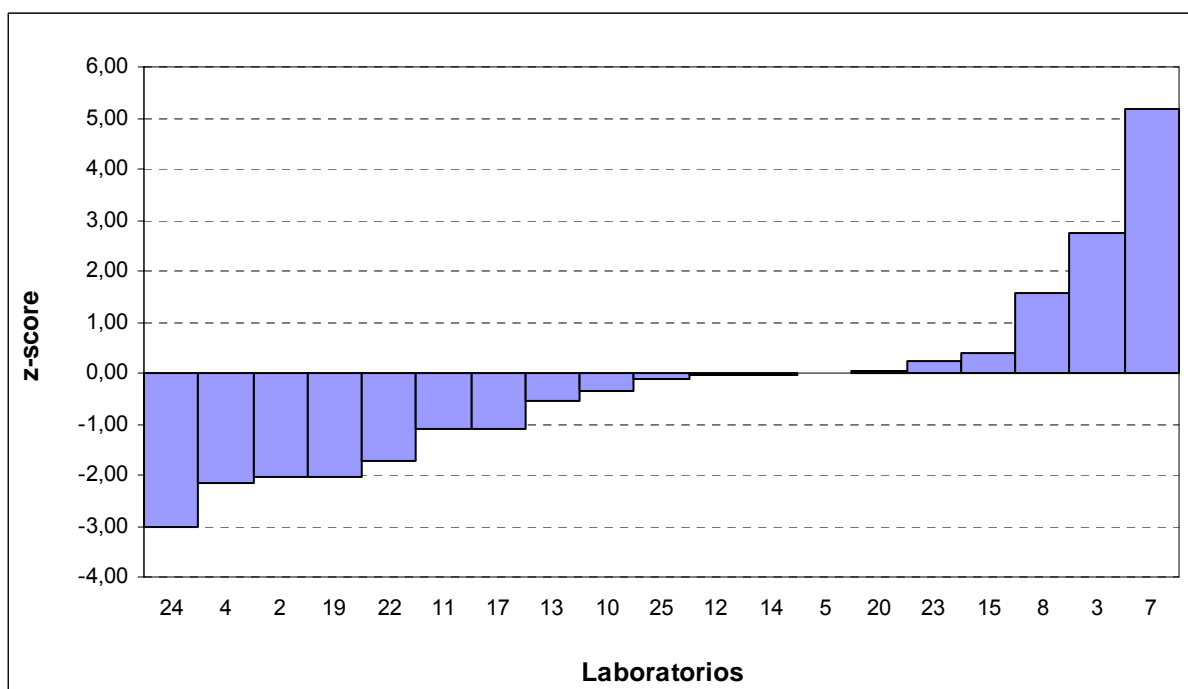
GRÁFICO 8 Parámetro z – Cromo
