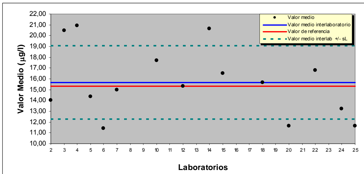
GRÁFICO 4 Datos enviados por los participantes – Mercurio
