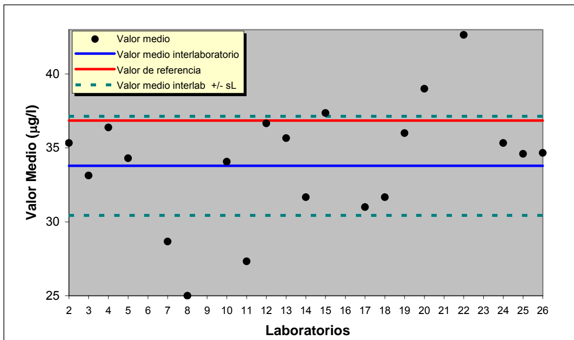
GRÁFICO 2 Datos enviados por los participantes - Cadmio
