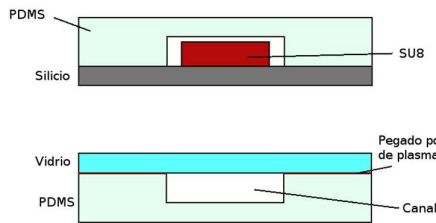
Fig. 3: Proceso de fabricación de un dispositivo microfluidico. Arr. Micromoldeado de PDMS con molde de SU8. Ab. Cerrado de las cavidades con portaobjeto de vidrio.
