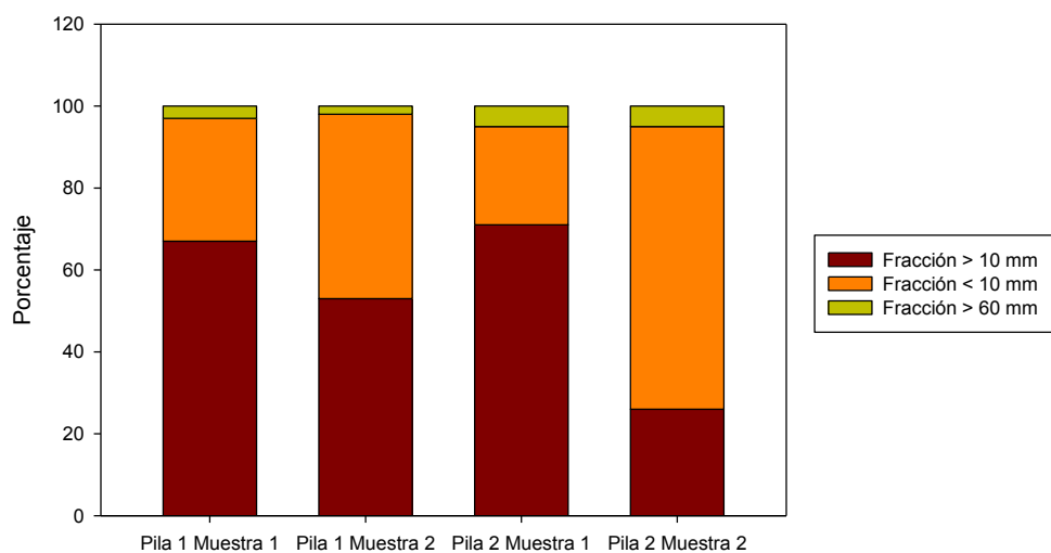
Figura: 13 Evolución en el tiempo del peso de cada fracción según su granulometría
