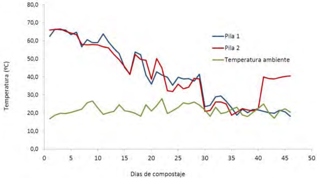
Figura 12 Evolución de la temperatura diaria
