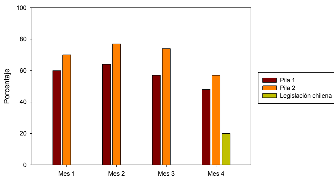
Figura 14 Evolución del Carbono Orgánico total (% en peso) a lo largo del tiempo comparado con los valores estipulados en la legislación chilena Nch 2280/04.
