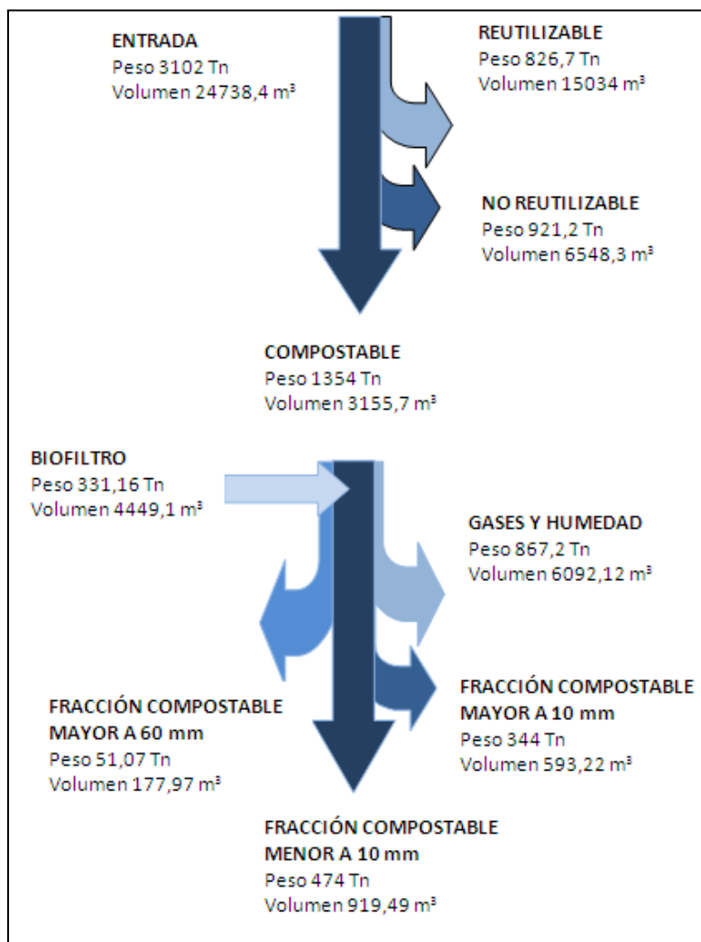
Figura 15 Balance de masa total para un año. Fuente: Elaboración propia
